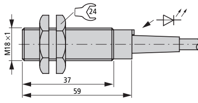
LSO-R18S-S300-LD
